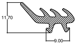
Die No. : 0-697 Wt/mtr : 110 gm/mtr
