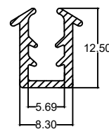
Die No. : 1059A Wt/mtr : 80 gm/mtr
