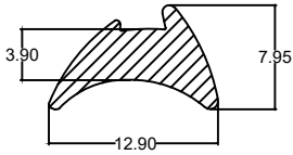
Die No. : 10316 Wt/mtr : 67 gm/mtr
