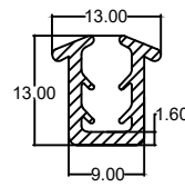
Die No. : 2030 Wt/mtr : 100 gm/mtr
