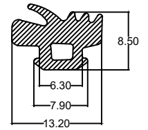
Die No. : 2064 Wt/mtr : 100 gm/mtr
