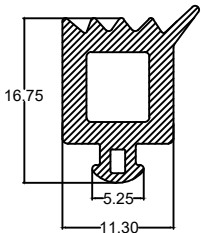
Die No. : 2211 Wt/mtr : 160 gm/mtr
