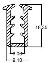
Die No. : 10263 Wt/mtr : 109 gm/mtr
