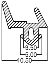
Die No. : 10095 Wt/mtr : 42 gm/mtr
