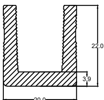
Die No. : 10421 Wt/mtr : 266 gm/mtr
