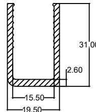
Die No. : 10034 Wt/mtr : 214 gm/mtr
