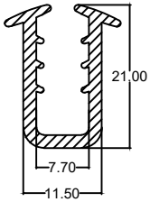
Die No. : 10292 Wt/mtr : 144 gm/mtr
