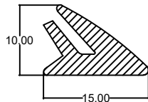
Die No. : 10178 Wt/mtr : 82 gm/mtr
