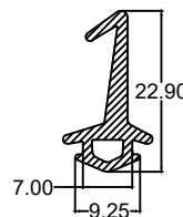
Die No. : 3363 Wt/mtr : 54 gm/mtr
