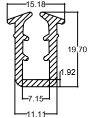
Die No. : 10064 Wt/mtr : 135 gm/mtr
