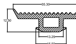
Die No. : 2412 Wt/mtr : 240 gm/mtr
