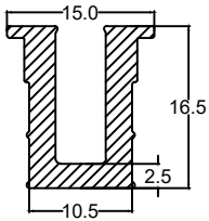
Die No. : 1046 Wt/mtr : 170 gm/mtr
