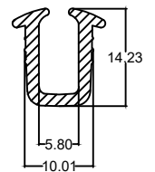
Die No. : 10165 Wt/mtr : 91 gm/mtr
