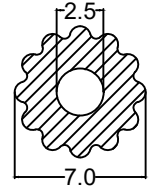
Die No. : 2234 Wt/mtr : 44 gm/mtr
