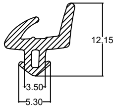
Die No. : 10150 Wt/mtr : 58 gm/mtr
