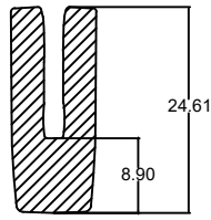
Die No. : 10252 Wt/mtr : 225 gm/mtr
