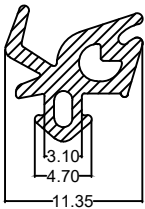
Die No. : 10175 Wt/mtr : 60 gm/mtr
