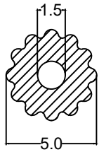
Die No. : 1818 Wt/mtr : 26 gm/mtr
