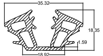
Die No. : 10193 Wt/mtr : 248 gm/mtr
