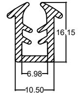
Die No. : 1027 Wt/mtr : 120 gm/mtr
