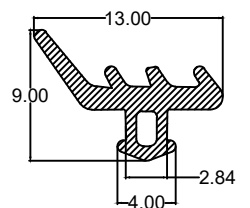
Die No. : 1876 Wt/mtr : 50 gm/mtr
