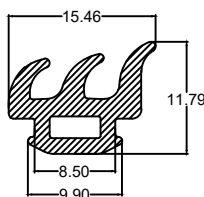
Die No. : 2381 Wt/mtr : 120 gm/mtr
