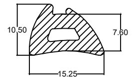
Die No. : 10131 Wt/mtr : 125 gm/mtr
