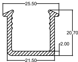
Die No. : 2236 Wt/mtr : 175 gm/mtr
