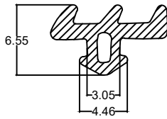
Die No. : 10099 Wt/mtr : 48 gm/mtr
