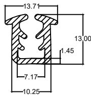
Die No. : 10104 Wt/mtr : 72 gm/mtr
