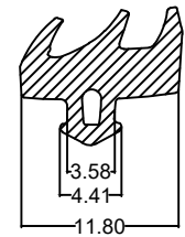
Die No. : 10311 Wt/mtr : 77 gm/mtr
