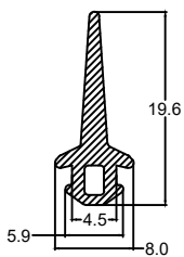
Die No. : 1714 Wt/mtr : 73 gm/mtr
