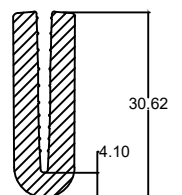
Die No. : 10226 Wt/mtr : 305 gm/mtr
