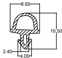
Die No. : 10257 Wt/mtr : 40 gm/mtr
