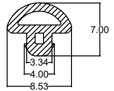
Die No. : 10118 Wt/mtr : 38 gm/mtr
