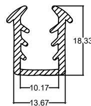
Die No. : 10297 Wt/mtr : 136 gm/mtr
