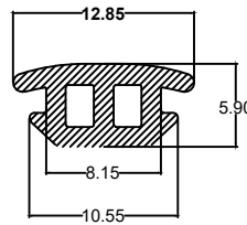
Die No. : 1900 Wt/mtr : 62 gm/mtr
