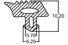
Die No. : 10013 Wt/mtr : 85 gm/mtr
