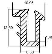
Die No. : 10396 Wt/mtr : 70 gm/mtr
