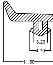
Die No. : 10048 Wt/mtr : 40 gm/mtr
