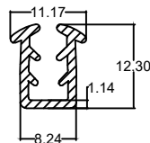
Die No. : 10142 Wt/mtr : 70 gm/mtr
