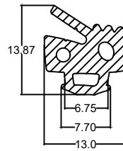
Die No. : 10038 Wt/mtr : 120 gm/mtr
