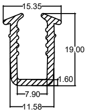
Die No. : 10065 Wt/mtr : 115 gm/mtr
