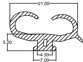
Die No. : 10044 Wt/mtr : 97 gm/mtr
