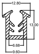
Die No. : 1480 Wt/mtr : 94 gm/mtr
