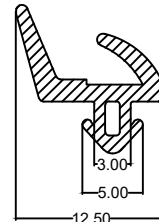
Die No. : 10020 Wt/mtr : 58 gm/mtr
