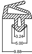
Die No. : 10021 Wt/mtr : 53 gm/mtr
