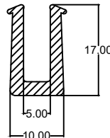
Die No. : 10221 Wt/mtr : 130 gm/mtr
