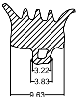
Die No. : 10231 Wt/mtr : 85 gm/mtr
