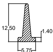
Die No. : 1187 Wt/mtr : 40 gm/mtr
