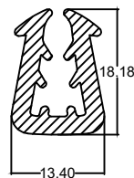
Die No. : 10197 Wt/mtr : 164 gm/mtr
