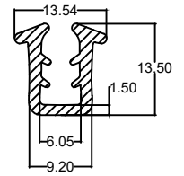
Die No. : 10134 Wt/mtr : 80 gm/mtr
