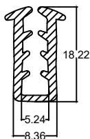
Die No. : 10166 Wt/mtr : 85 gm/mtr
