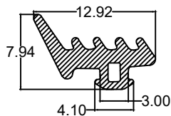
Die No. : 3330 Wt/mtr : 55 gm/mtr
