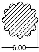
Die No. : 1785 Wt/mtr : 39 gm/mtr
