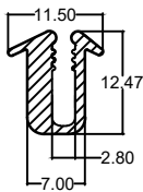
Die No. : 10298 Wt/mtr : 75 gm/mtr
