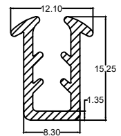
Die No. : 10181 Wt/mtr : 87 gm/mtr
