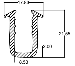
Die No. : 10291 Wt/mtr : 134 gm/mtr
