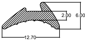
Die No. : 1423 Wt/mtr : 38 gm/mtr
