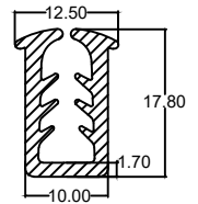
Die No. : 2255A Wt/mtr : 142 gm/mtr
