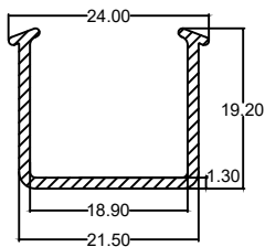
Die No. : 10140 Wt/mtr : 54 gm/mtr
