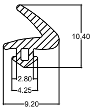
Die No. : 1533 Wt/mtr : 50 gm/mtr
