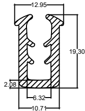
Die No. : 10317 Wt/mtr : 140 gm/mtr
