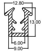
Die No. : 1479 Wt/mtr : 90 gm/mtr
