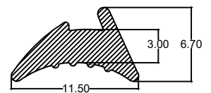
Die No. : 1163 Wt/mtr : 61 gm/mtr
