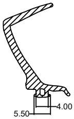
Die No. : 10074 Wt/mtr : 158 gm/mtr
