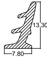
Die No. : 10103 Wt/mtr : 50 gm/mtr
