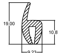
Die No. : 10264 Wt/mtr : 113 gm/mtr
