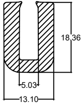
Die No. : 10237 Wt/mtr : 219 gm/mtr
