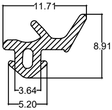
Die No. : 10174 Wt/mtr : 40 gm/mtr
