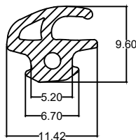
Die No. : 10147 Wt/mtr : 68 gm/mtr
