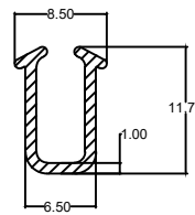
Die No. : 10145 Wt/mtr : 39 gm/mtr
