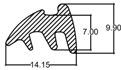
Die No. : 1532 Wt/mtr : 96 gm/mtr
