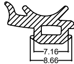
Die No. : 10087 Wt/mtr : 73 gm/mtr
