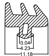
Die No. : 10310 Wt/mtr : 64 gm/mtr
