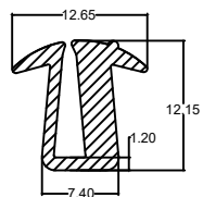
Die No. : 10387 Wt/mtr : 76 gm/mtr
