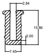
Die No. : 10222 Wt/mtr : 122 gm/mtr
