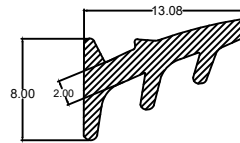
Die No. : 10141 Wt/mtr : 63 gm/mtr
