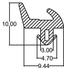
Die No. : 10216 Wt/mtr : 55 gm/mtr
