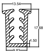
Die No. : 10443 Wt/mtr : 124 gm/mtr
