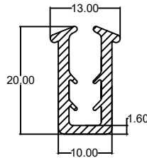
Die No. : 1530A Wt/mtr : 124 gm/mtr
