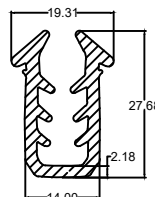
Die No. : 10465 Wt/mtr : 243 gm/mtr
